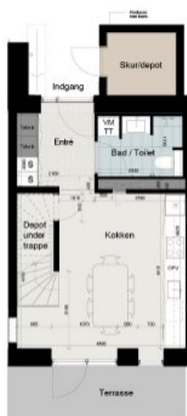
STUEPLAN
